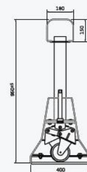
SECCIÓN ESTÁNDAR
